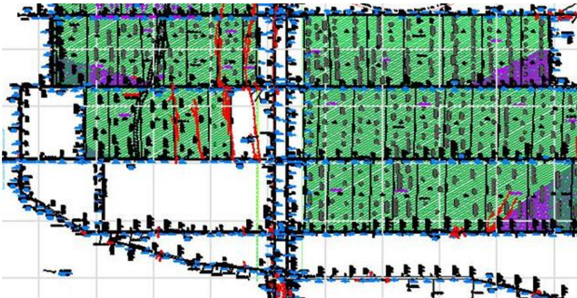
Rys. 3. Geolisp umożliwia wektoryzację wszelkich map górniczych.
