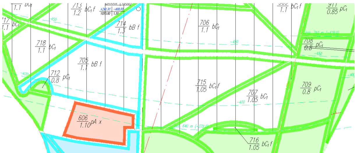
Rys. 6. Program kontroluje topologię parcel i oblicza im średnią miąższość na podstawie numerycznego modelu złoża.
