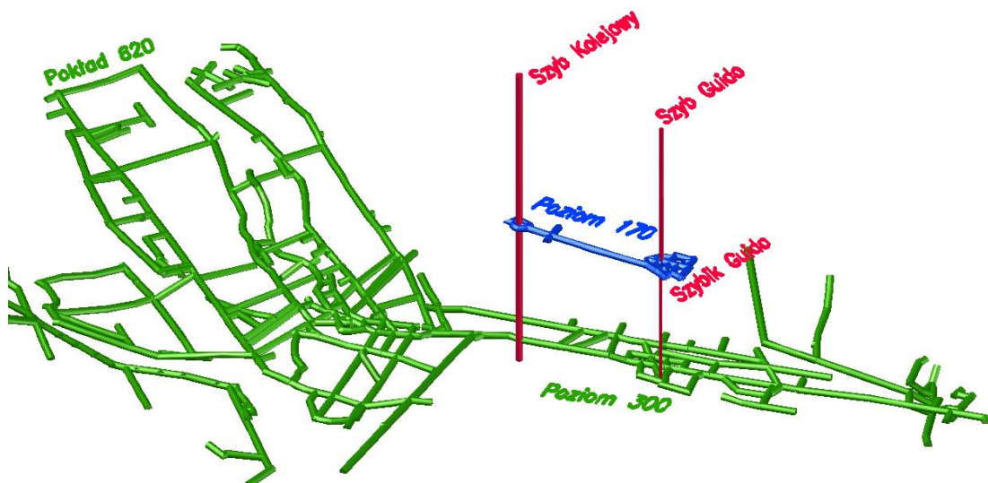
Rys. 5. Model przestrzenny wyrobisk górniczych.
